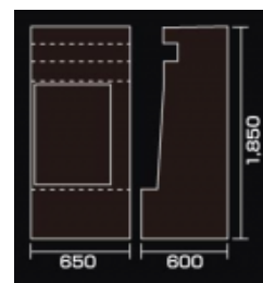
外形寸法:W650×D600×H1850 使用電源:AC100V(50Hz/60Hz)
